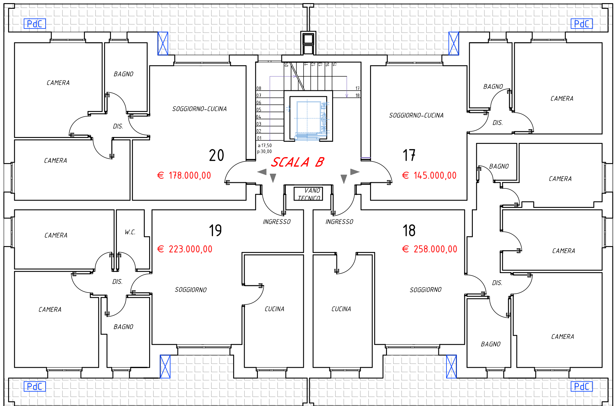
Pianta piano quarto - scala B
