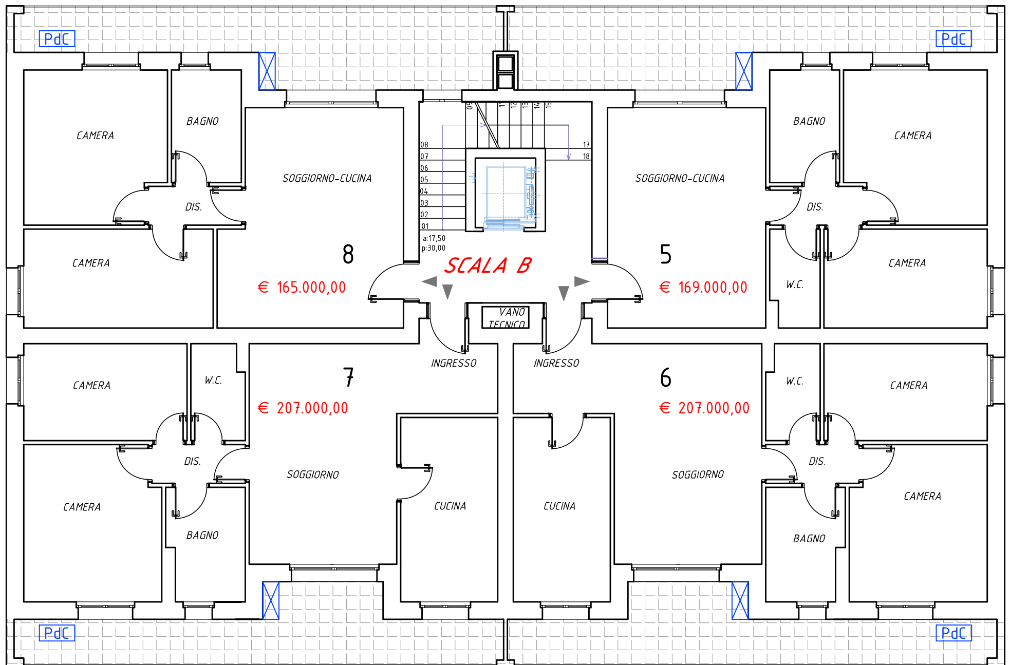
Pianta piano primo - scala B
